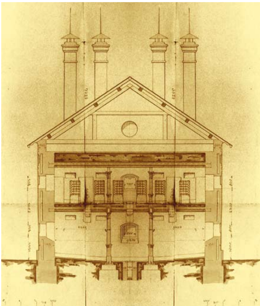
Chłodnia dla rzeźni miejskiej, projekt 1897. (fot. Archiwum Państwowe w Katowicach, Oddział w Cieszynie)
